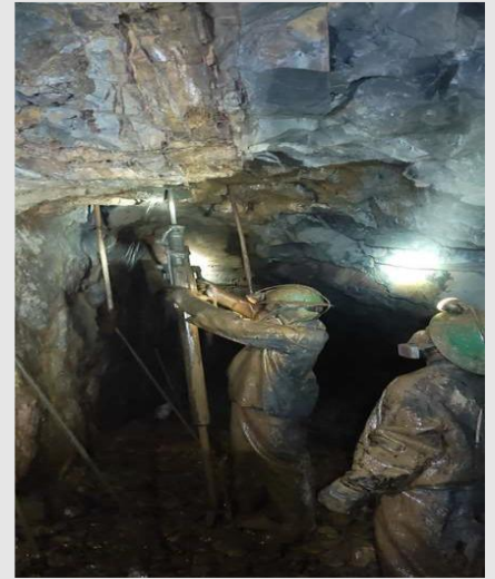
AVANCE CHIMENEA CONVENCIONAL
