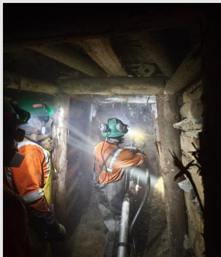
AVANCE JACKLEG SECCION 2.4 X 2.4 M
