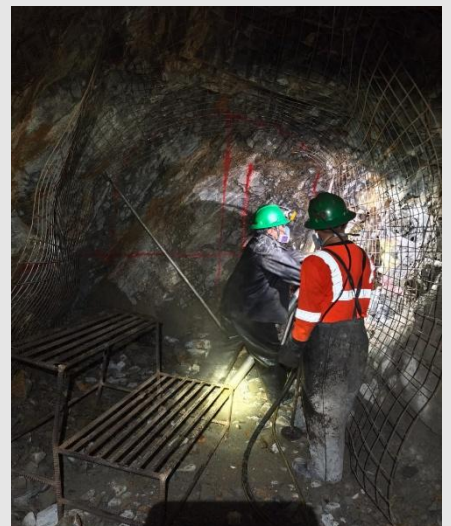
SOSTENIMIENTO CON PERNOS Y MALLA
