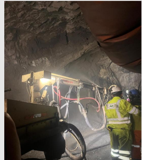
LANZADO DE SHOTCRETE EN VIA HUMEDA
